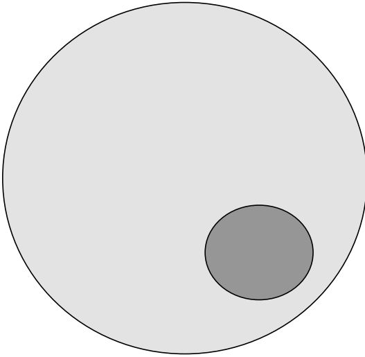
Abbildung 1: Die dunklere Menge ist Teilmenge der helleren. Beide Mengen enthalten unendlich und gleich viele Punkte.
