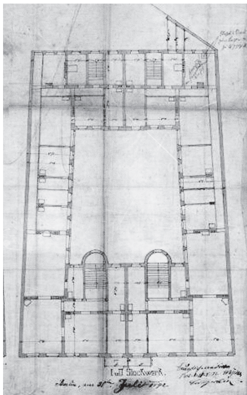
Abb. 10: «Die Räume brachen im rechten Winkel»: Grundriss des 1. und 2. Stockwerks im Haus Kronprinzenufer 5
