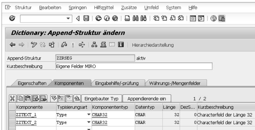
Abbildung 6.2 Append-Struktur ZZRSEG
