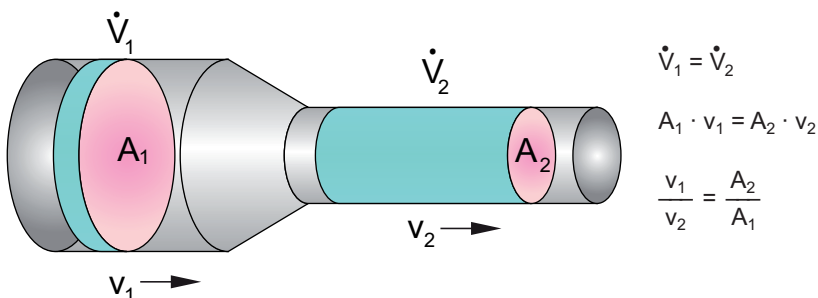
Abbildung 1-5 Kontinuitätsgleichung
