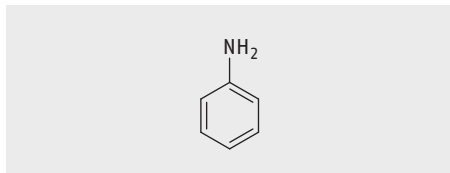
• Abb. 6.1 Strukturformel von Anilin
