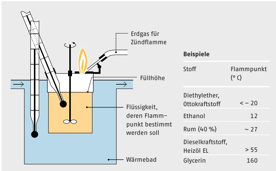
● Abb. 1.3 Flammpunktbestimmung nach BG RCI (Berufsgenossenschaft Rohstoffe und chemische Industrie, http://www.gischem.de )
