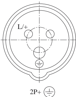
Bild 9.4 Anschlussbelegung von dreipoligen Industriesteckdosen (Skizze Mennekes)
