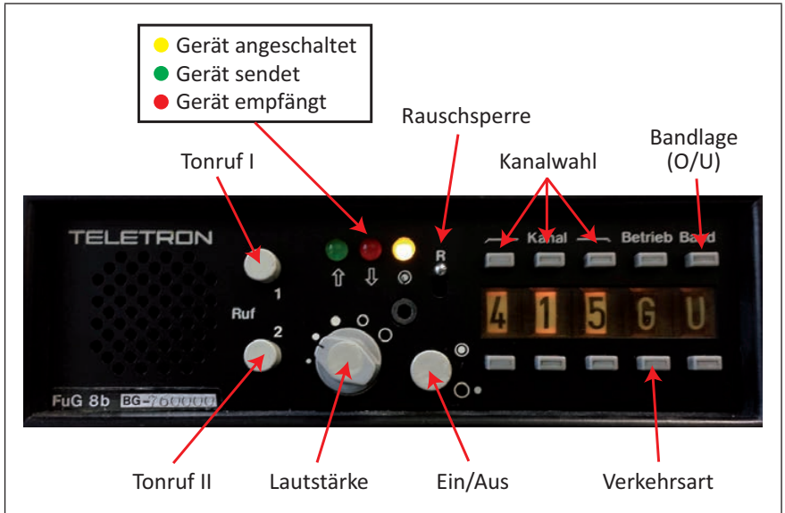
Abbildung 8: FuG 8b-1 (Quelle: Verfasser)
