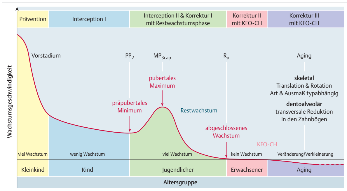
Abb. 4.2 Kieferorthopädisches Timing in Abhängigkeit der Wachstumskurve nach Björk [213], [214], ergänzt um den Zeitraum des Agings.
