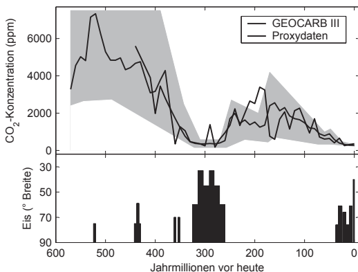
Abb. 1.2: Verlauf von \text{CO}_2 -Konzentration und Klima über die abgelaufenen 600 Millionen Jahre. Die schwarze Kurve zeigt eine Rekonstruktion aus vier unabhängigen Typen von Proxy-Daten. Die graue Kurve (mit dem grauen Unsicherheitsbereich) ergibt sich aus einer Modellsimulation des Kohlenstoffkreislaufs. Der untere Teil der Grafik zeigt, als Hinweis auf das Klima, bis zu welchem Breitengrad Kontinental-Eis auf der Erde vorgedrungen ist. Phasen mit niedrigem \text{CO}_2 -Gehalt der Atmosphäre fallen mit Vereisungsphasen zusammen. (Quelle: Royer et al. 2004 10 )
