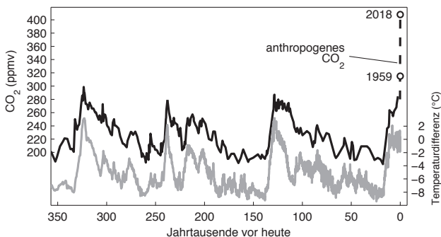
Abb. 1.1: Verlauf der Temperatur in der Antarktis (graue Kurve, Änderung relativ zu heute) und der \text{CO}_2 -Konzentration der Atmosphäre (schwarze Kurve) über die abgelaufenen 350 000 Jahre aus dem Wostok-Eiskern. 7 Man erkennt drei Eiszeitzyklen. Am Ende ist der vom Menschen verursachte Anstieg des \text{CO}_2 gezeigt.
