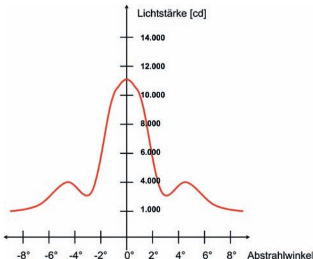
Bild 3: Lichtstärkenverteilungskurve
