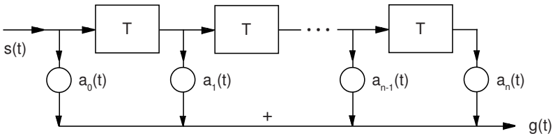
Abb. 5.10. Zeitvariantes Transversalfilter
