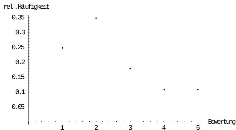
Kap. 2 Abbildung 1 - Häufigkeitsfunktion einer Beliebtheitsfrage
