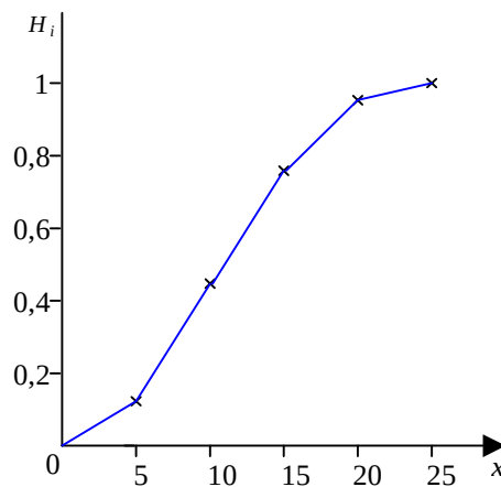
Kap.2 Abbildung 4 - Summenhäufigkeitspolygon der klassierten Daten zu den zurückgelegten Haltestellen aus Beispiel 3
