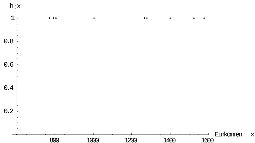
Kap.2 Abbildung 5 - Häufigkeiten selten auftretender Merkmalsausprägungen aus Beispiel 4
