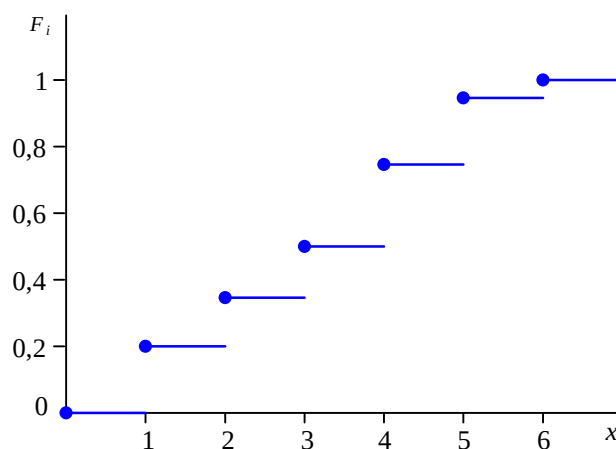
Kap.2 Abbildung 3 - Treppenfunktion zur Häufigkeitsverteilung der Schulnoten aus Beispiel 1
