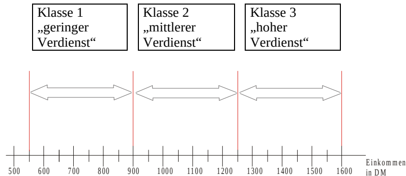
Kap.2 Abbildung 6 - Die Klassifizierung der Skala in einem Beispiel
