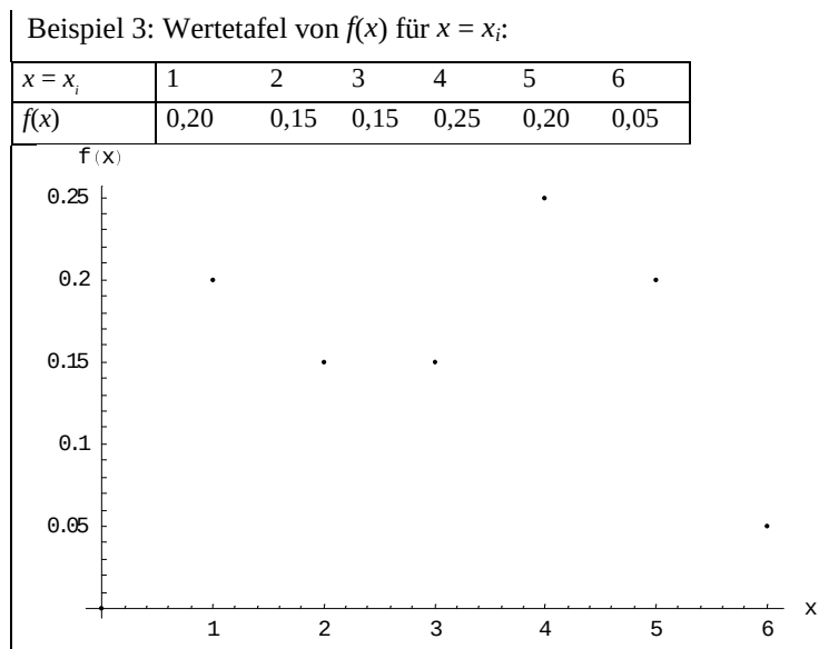
Kap.2 Abbildung 2 - Funktionsgraph der Häufigkeitsfunktion f(x) für die Schüler der 8. Klasse
